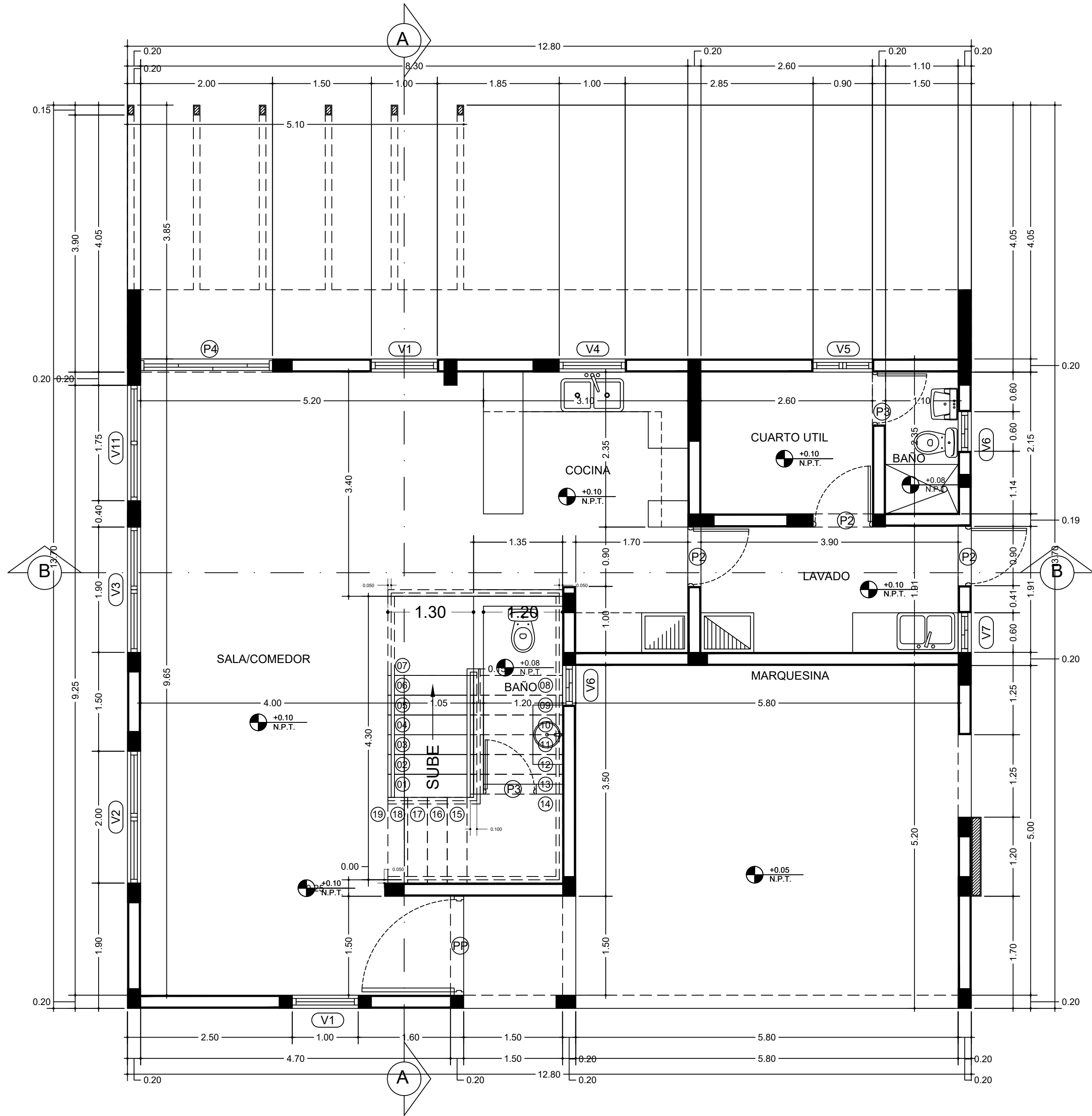
PLANTA ARQUITECTONICA DIMENSIONADA 1ER NIVEL - Esc. 1:50
