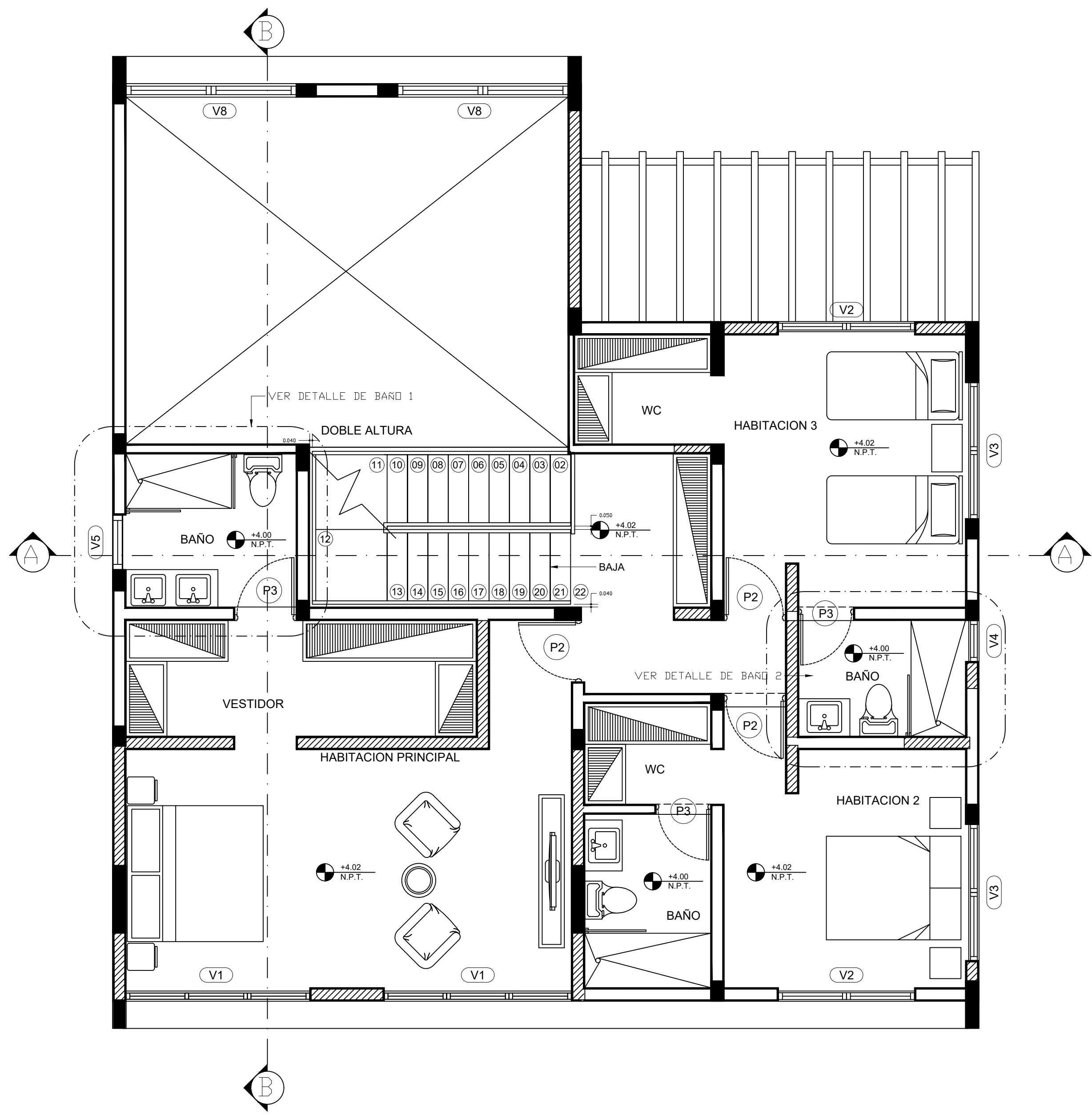
Planta Arquitectónica 2do nivel Esc. 1:50
